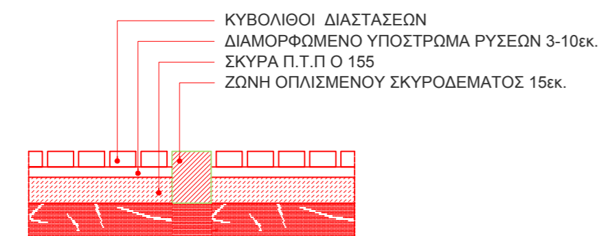
ΤΟΜΗ 1:20 ΣΗΜΕΙΟ ΑΛΛΑΓΗΣ ΚΥΒΟΛΙΘΩΝ
