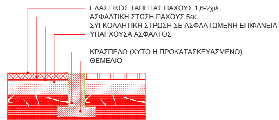
ΤΟΜΗ 1:20 ΓΗΠΕΔΟ ΣΕ ΑΣΦΑΛΤΩΜΕΝΗ ΕΠΙΦΑΝΕΙΑ ΣΕ ΕΠΑΦΗ ΜΕ ΔΑΠΕΔΟ ΑΠΟ ΚΥΒΟΛΙΘΟΥΣ
