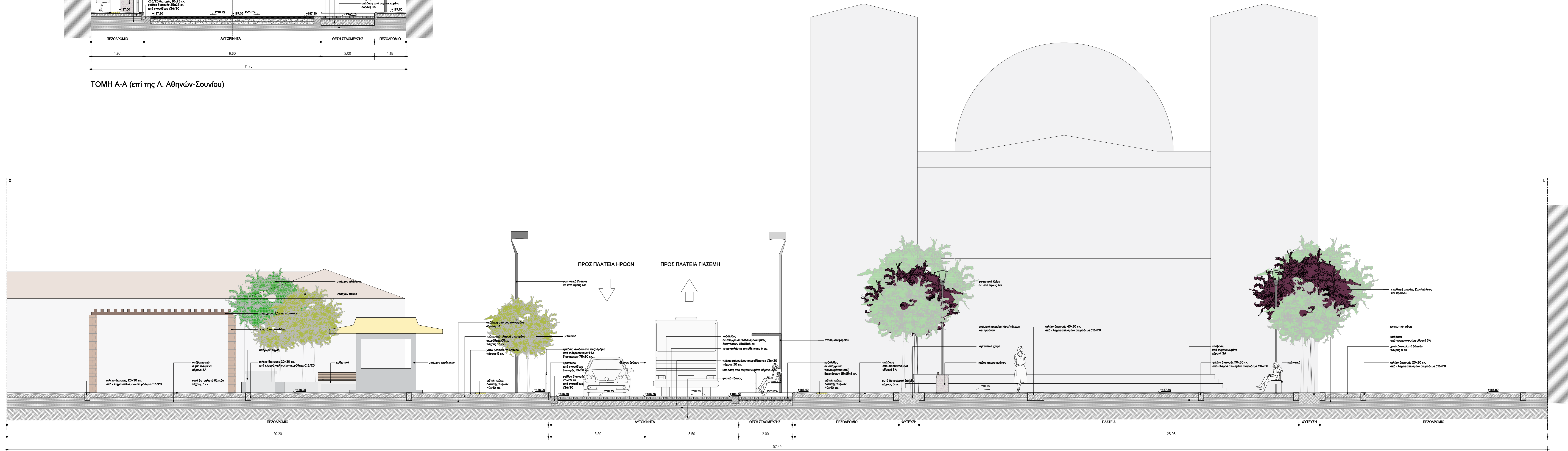
ΤΟΜΗ Β-Β (επί της Λ. Αθηνών-Σουνίου)
