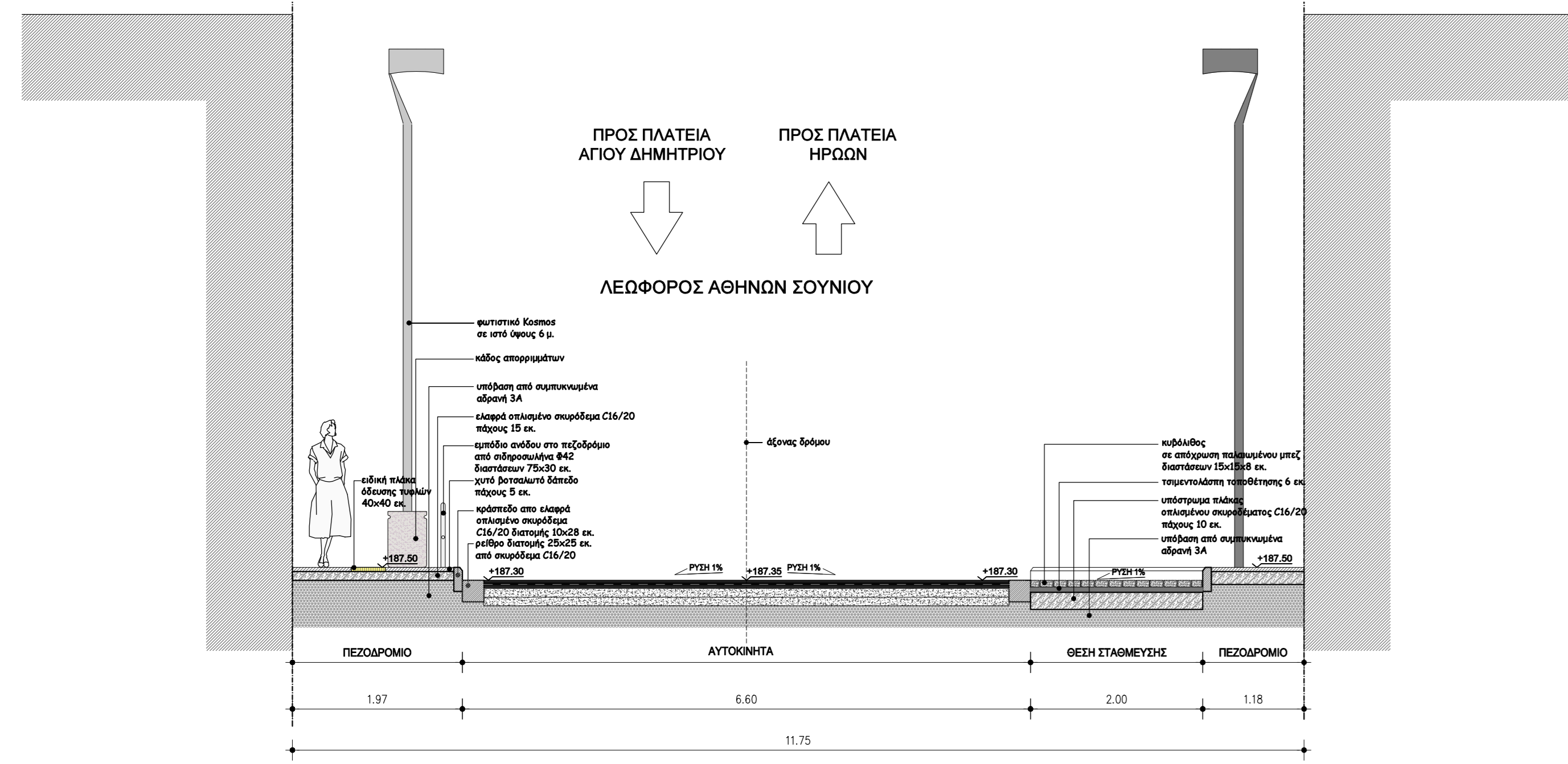
ΤΟΜΗ Α-Α (επί της Λ. Αθηνών-Σουνίου)
