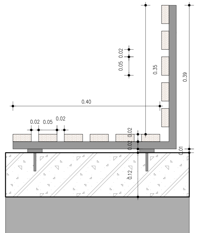
ΤΟΜΗ Α-Α ΚΛΙΜΑΚΑ 1:5
